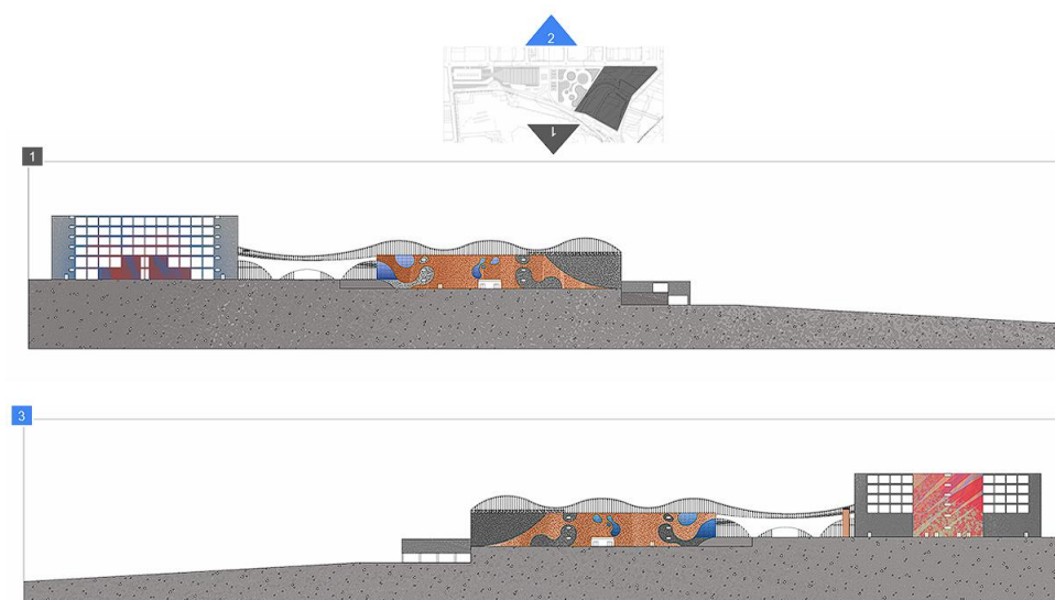
FIGURA 4 – Elevações laterais cultural Saraceni.
